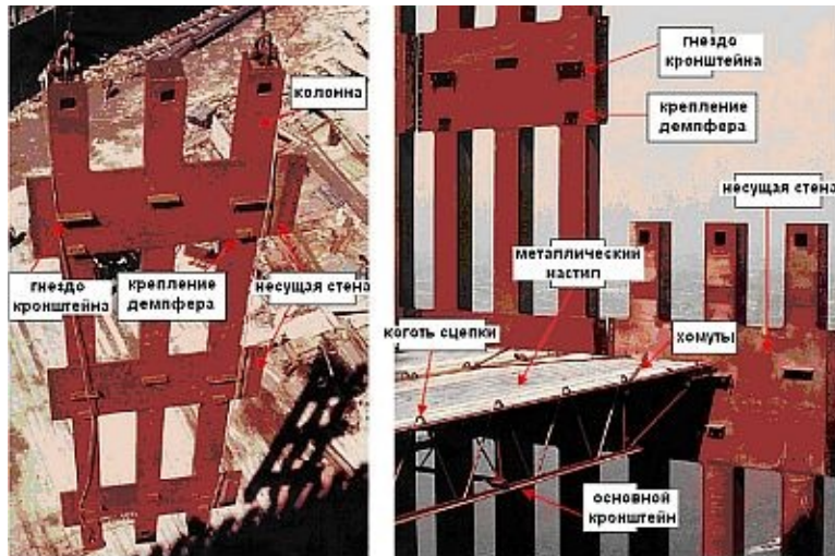
Figure 1-4. Perimeter column/spandrel assembly and floor structure. Структура сборок периферийных колонн/несущих стен и этажей.
